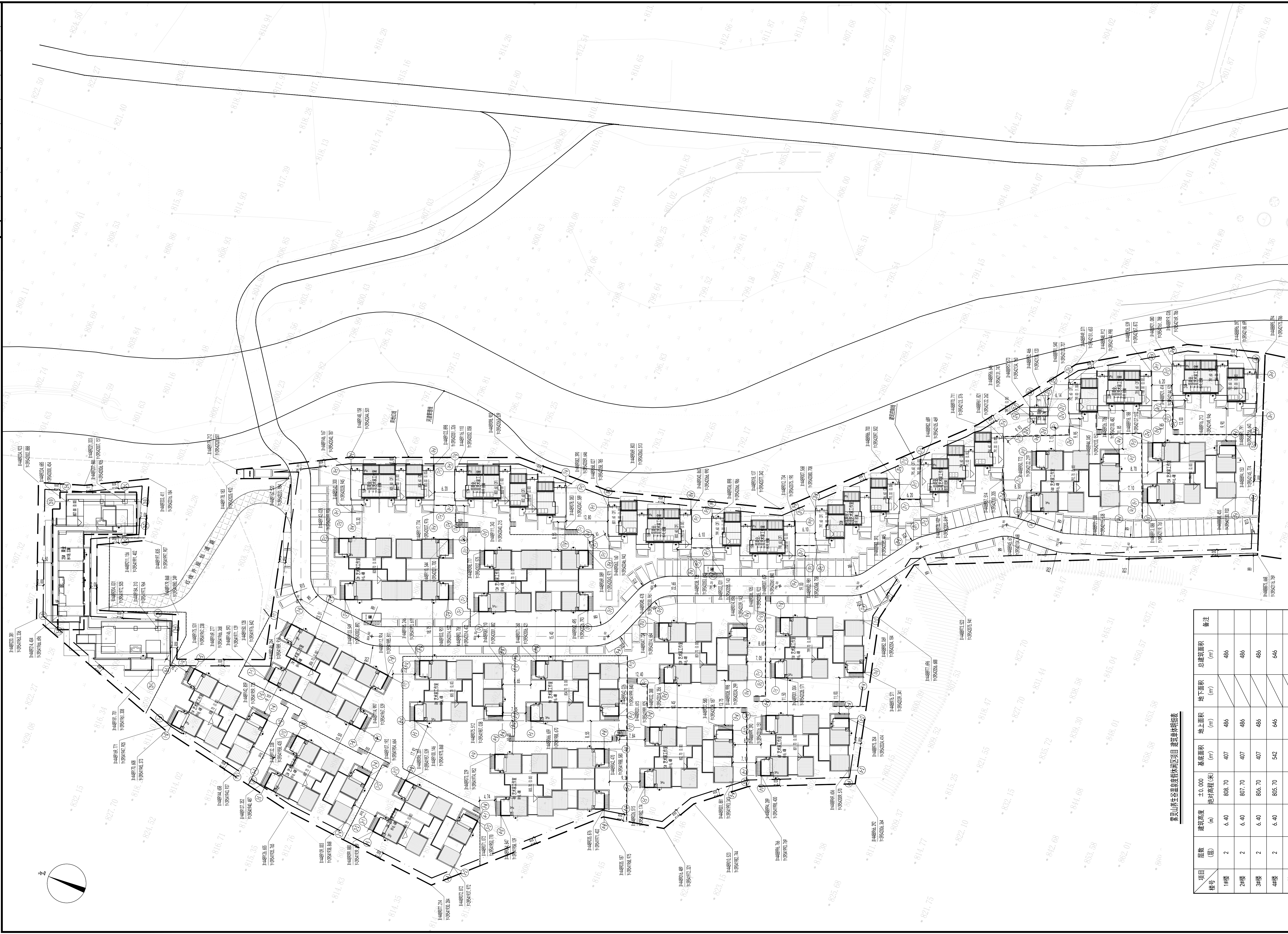
总平面图 1:500
